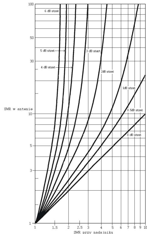
Rysunek 2 - Wykres pokazujący faktyczny SWR w antenie oparty o mierzony SWR przy nadajniku z stratami
